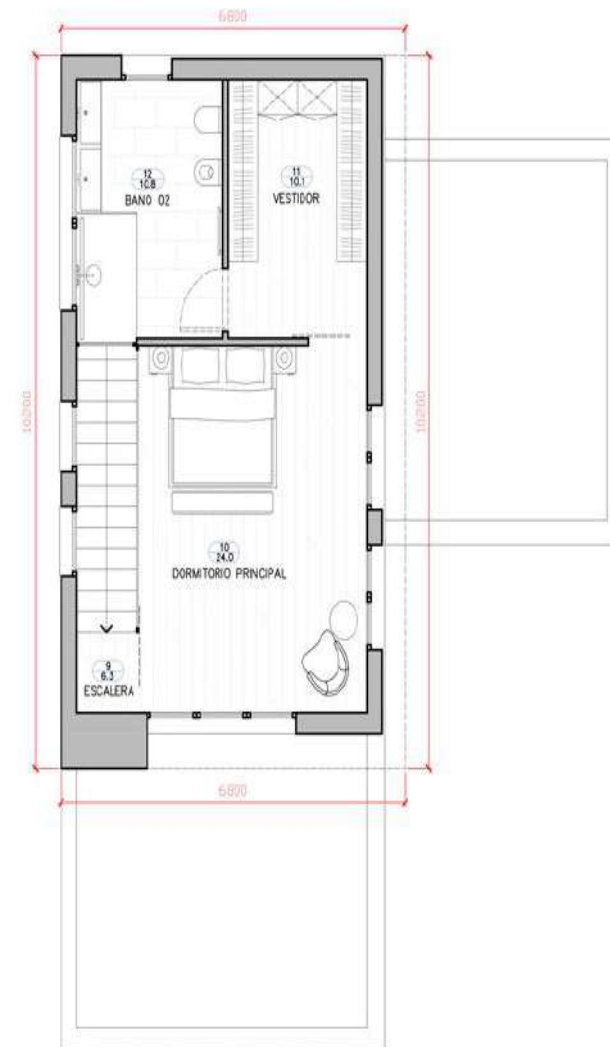
Primera Planta
