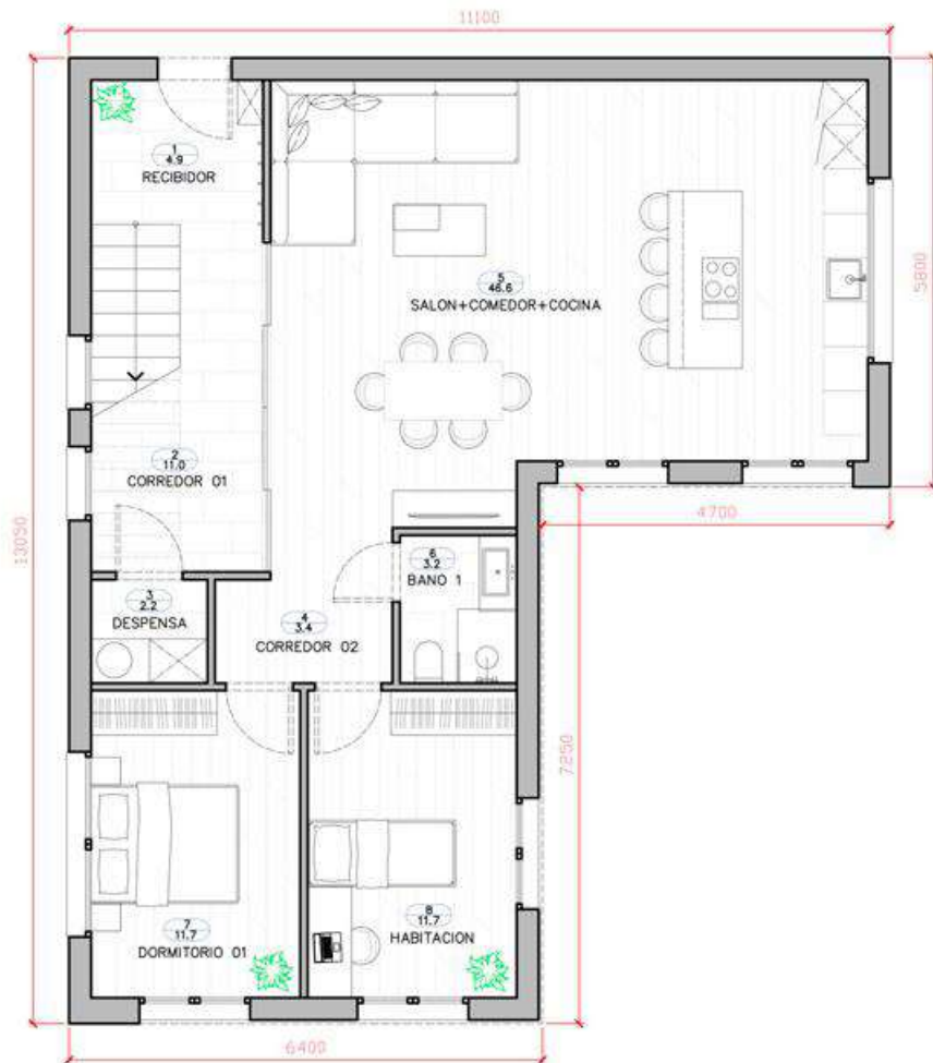
Planta Baja
