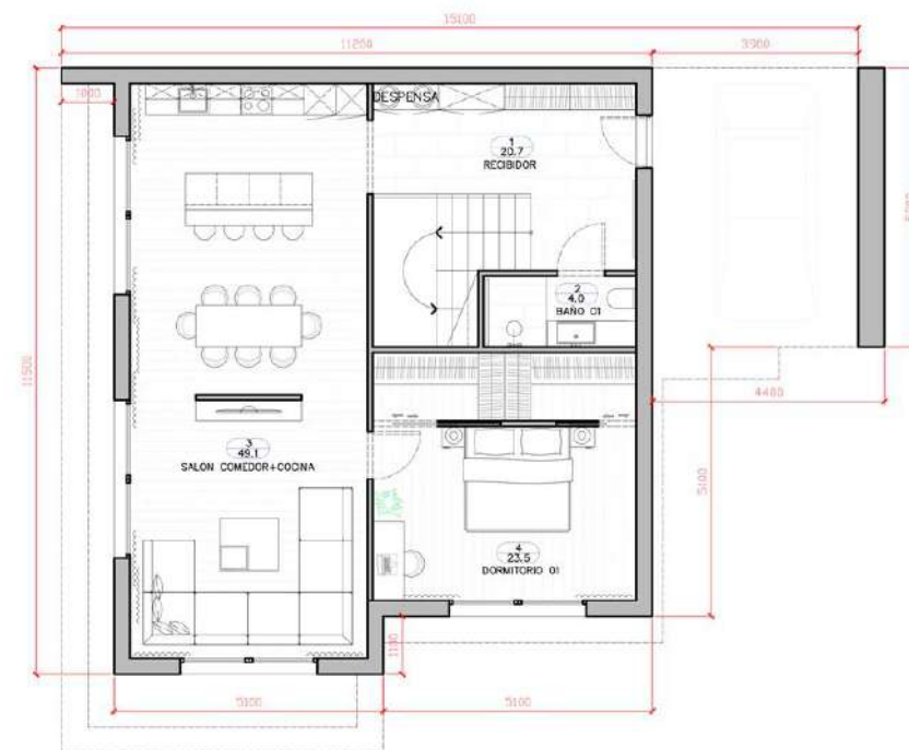
Primera Planta
