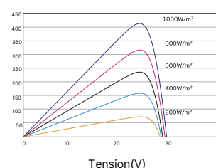
Courbes P-V du Module PV (420W)
