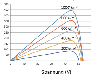
P-V-Kurven des PV-Moduls (445W)
