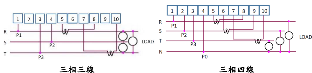
圖 6.1 接線圖
