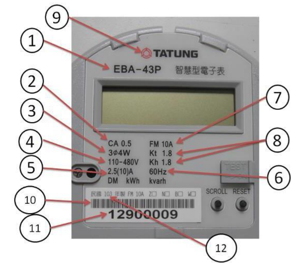
圖 3.1 銘板說明圖
