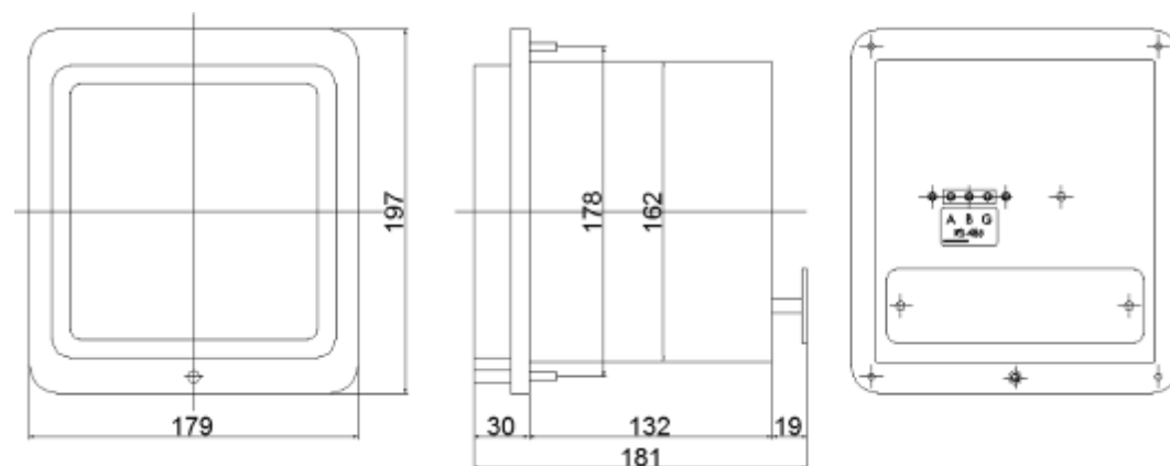
圖 2.1 電表外觀尺寸圖
