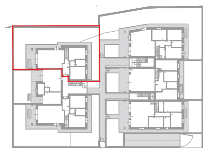
PLANIMETRIA GENERALE - Piano terra
