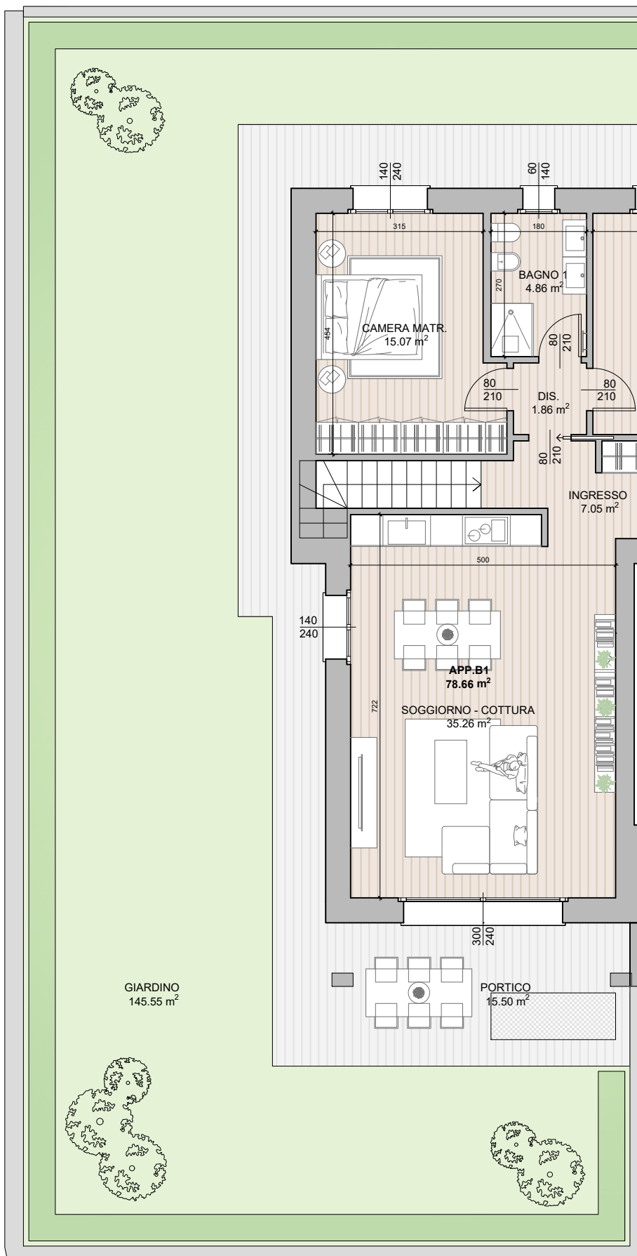
PIANO TERRA - appartamento B1
