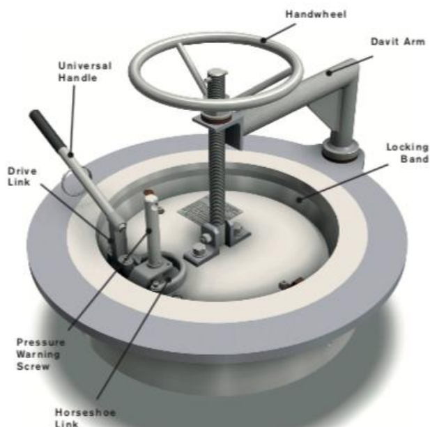
立式盲板（带吊臂）
