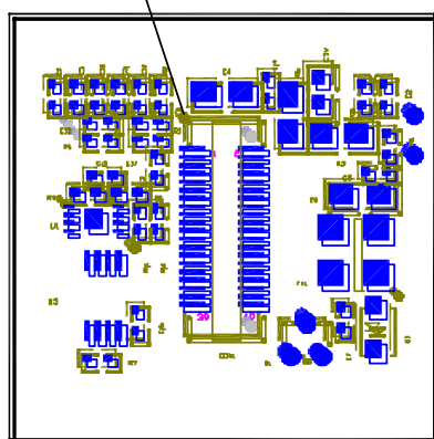
Pin_1 Mark
