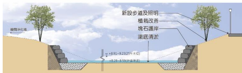
九番埤改善斷面
