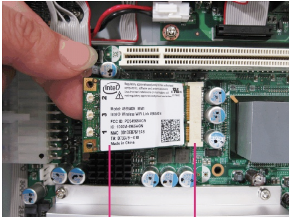
PCIe WiFi module
