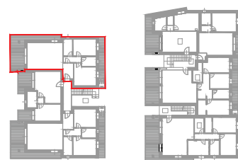
PLANIMETRIA GENERALE - Piano primo
