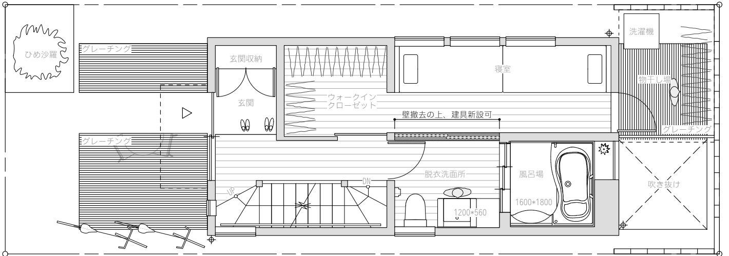
1階平面図
