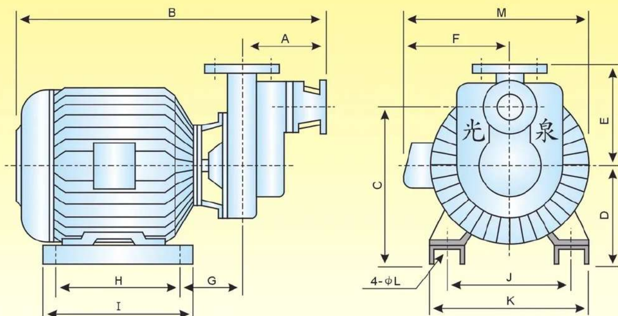
2P(2極)三相外觀尺寸圖
