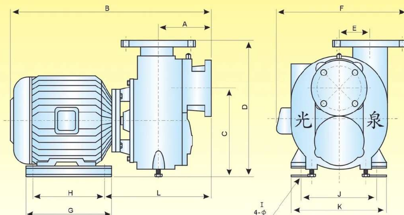
4P(4極)三相外觀尺寸圖
