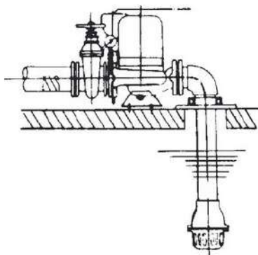
橫裝給水用 Horizontal Mounting
