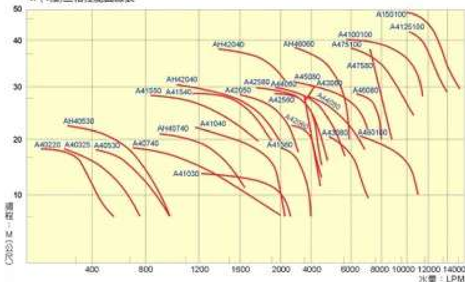
4P(4極)三相性能表[60Hz(1750R.P.M.)]
