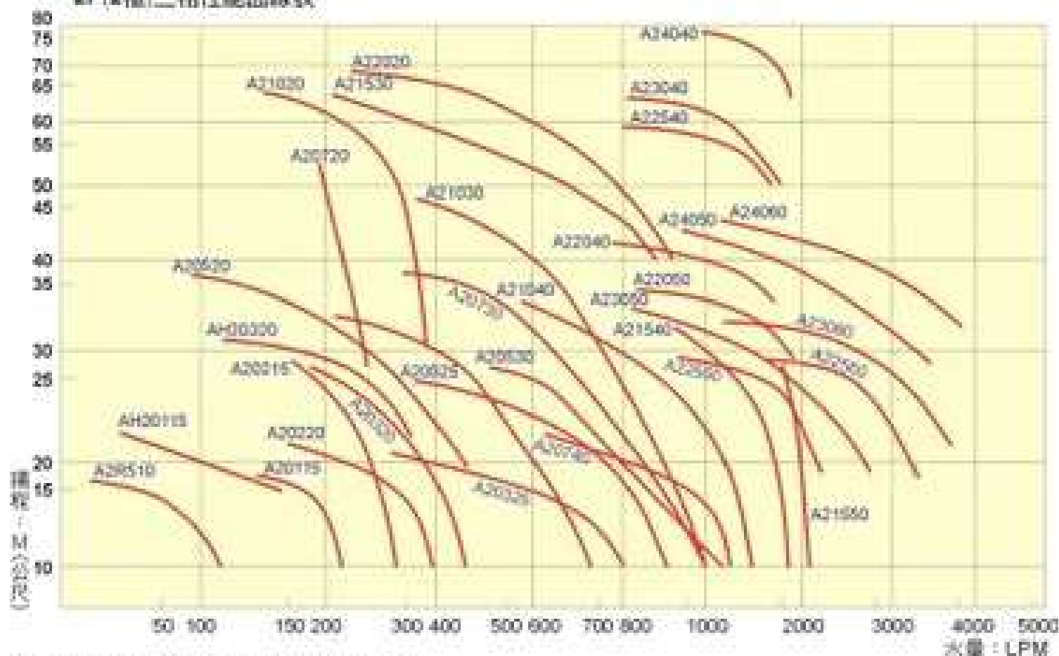
2P(2相)三相性能表(60Hz/3500R.P.M.)
