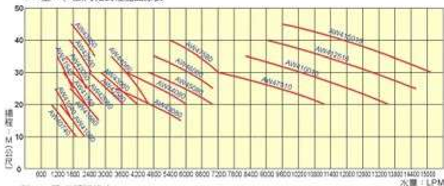
AW型4P(4極)三相性能表(60Hz(3500R.P.M.))
