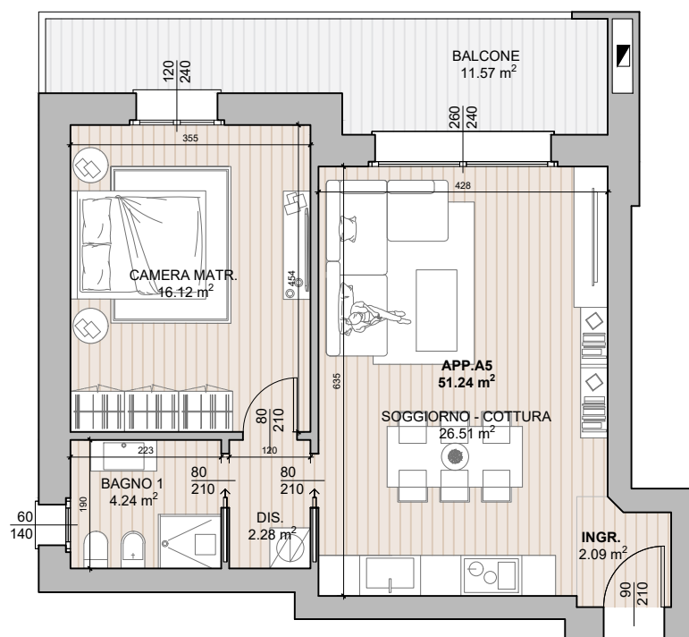
PIANO PRIMO - appartamento A5
