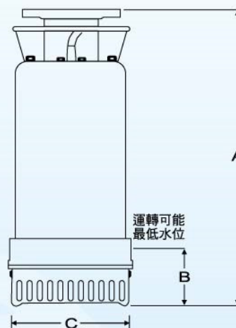
水陸兩用泵浦尺寸圖
