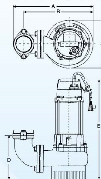
泛用型污水泵浦尺寸圖
