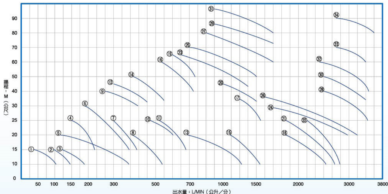
高性能聯軸渦卷泵浦三相性能規格表
