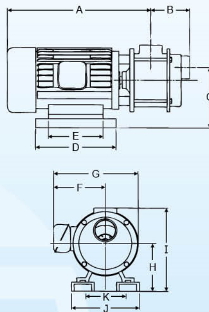
不銹鋼多段自吸式泵浦尺寸圖
