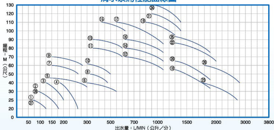
清水泵浦性能曲線圖
