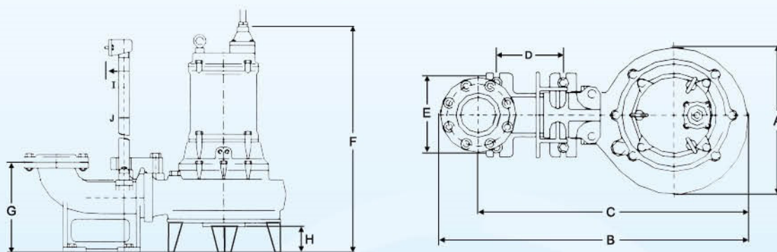
CBPT型 外型尺寸圖
