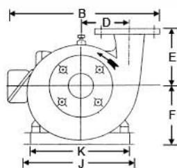
2P聯軸渦卷泵浦外型尺寸圖
