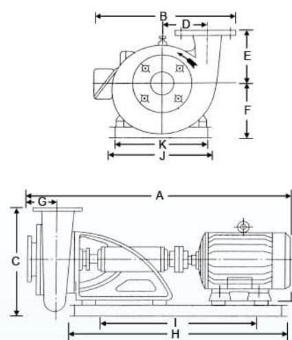
聯軸低噪音渦卷泵浦尺寸圖
