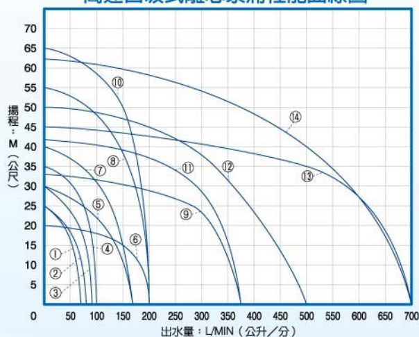
高速自吸式離心泵浦性能曲線圖
