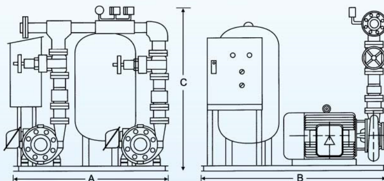
雙台交互並列隔膜式加壓機尺寸圖
