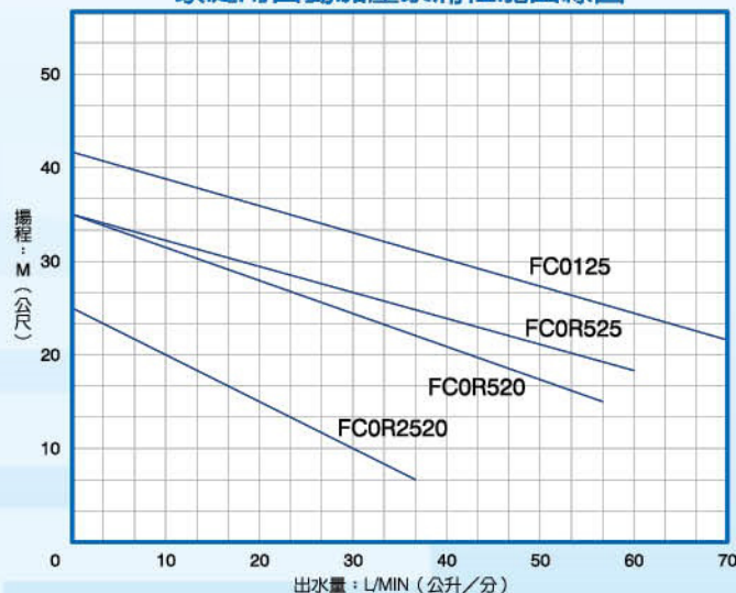
家庭用自動加壓泵浦性能曲線圖
