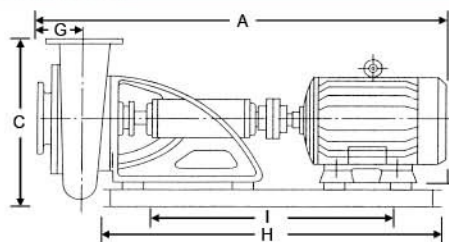
聯軸渦卷泵浦尺寸圖
