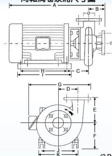
同軸渦卷泵浦尺寸圖
