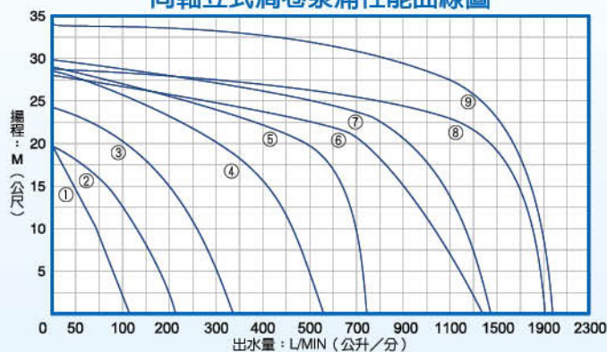
同軸立式渦卷泵浦性能曲線圖
