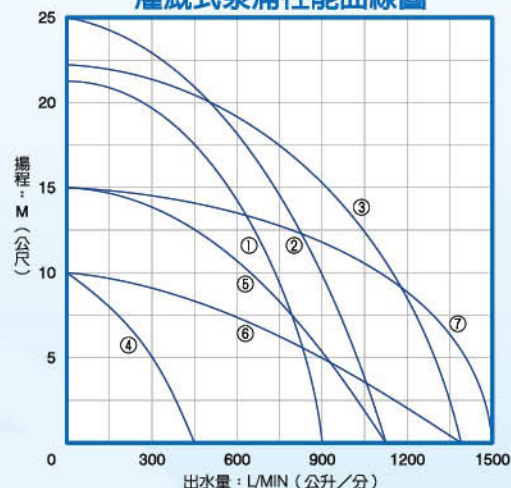
灌溉式泵浦性能曲線圖
