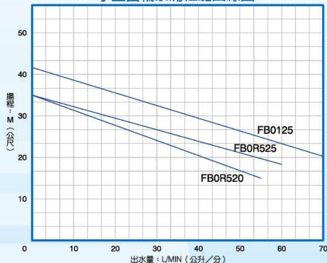
小型齒輪泵浦性能曲線圖
