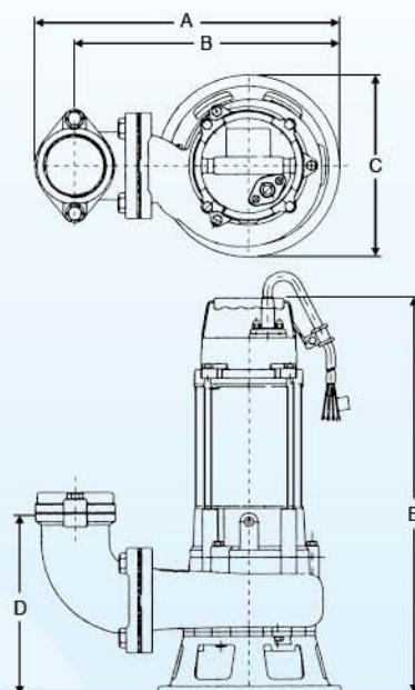
泛用型污物泵浦尺寸圖
