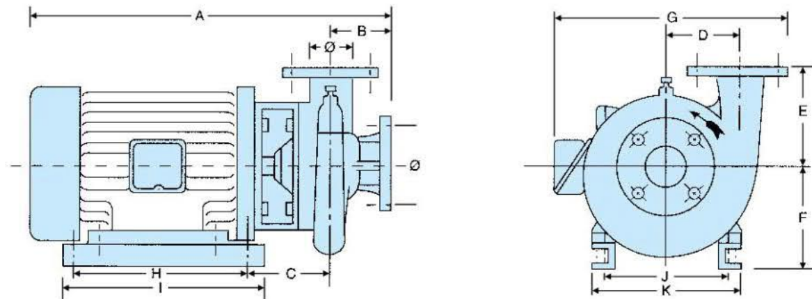
4P 同軸低噪音渦卷泵浦外型尺寸圖
