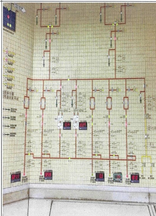
照片內容:變頻器系統單機模式 位 置:北放流站中控室
