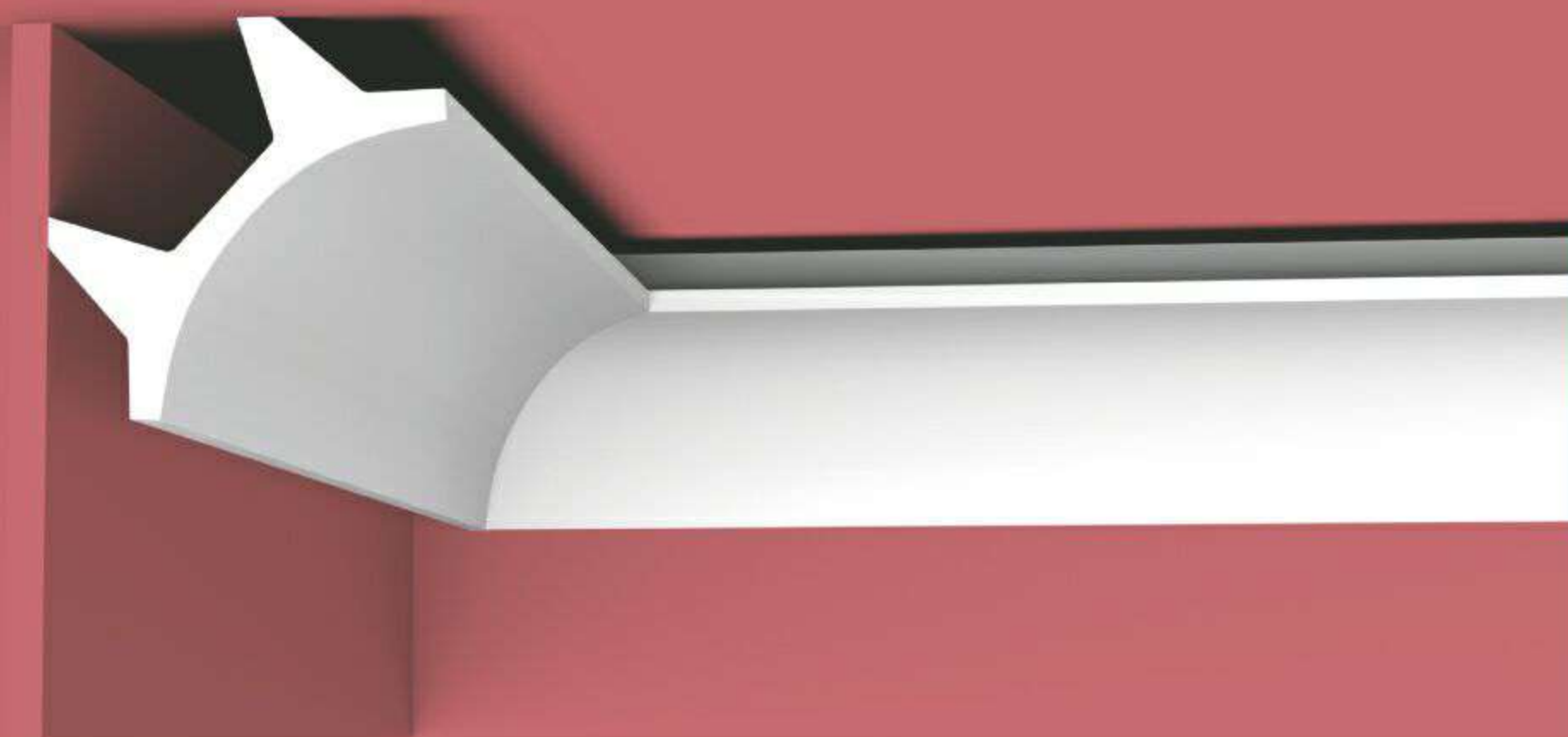
XT-9317 Height x Width x Length 高度 x 宽度 x 长度 90 x 90 x 2400 mm 90 = 130mm 90 90
