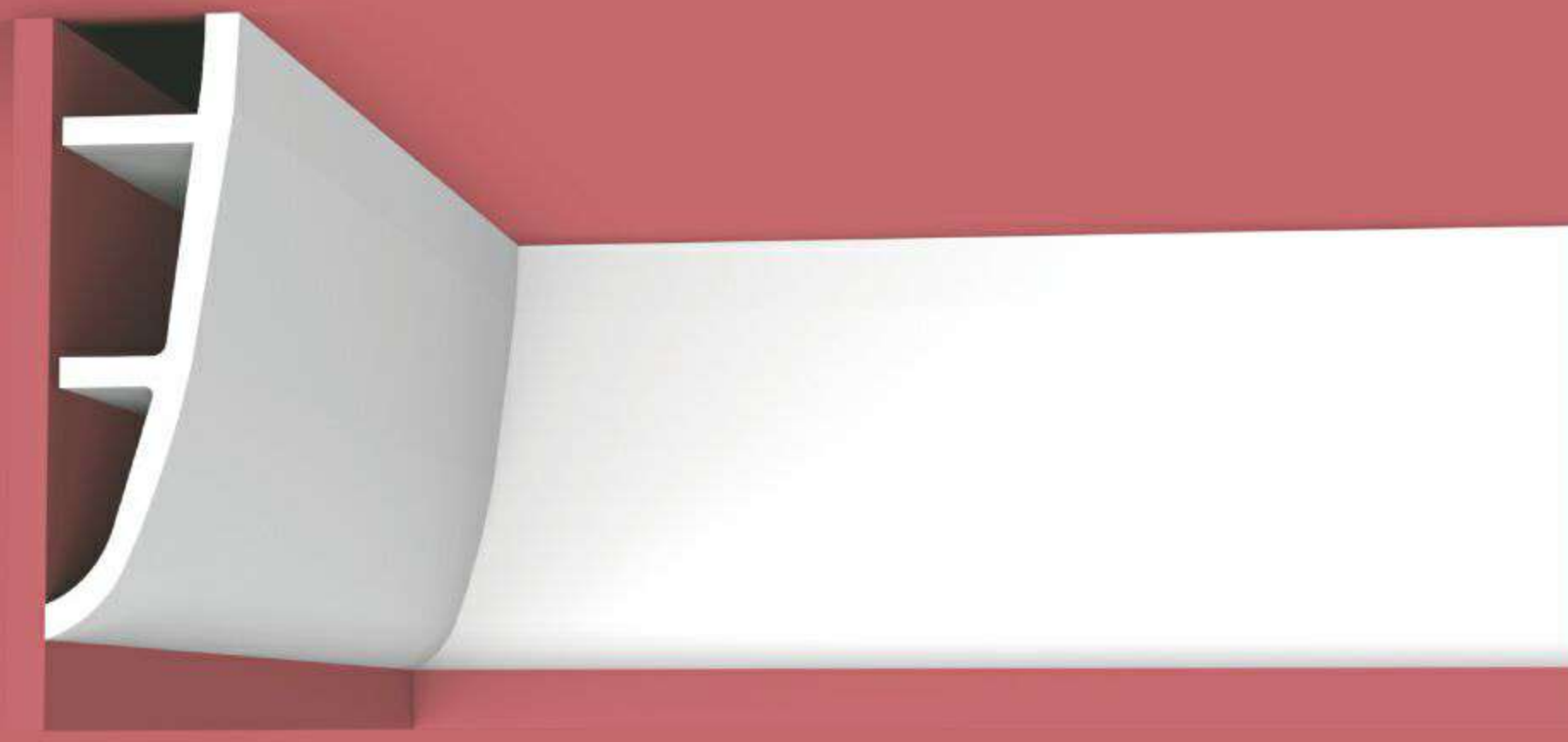
XT-9356 Height x Width x Length 高度 x 宽度 x 长度 180 x 50 x 2400 mm 50 180 185 mm
