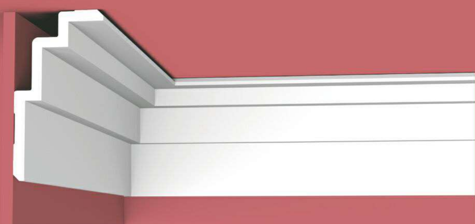
XT-9359 Height x Width x Length 高度 x 宽度 x 长度 190 x 100 x 2400 mm 100 190 200 mm
