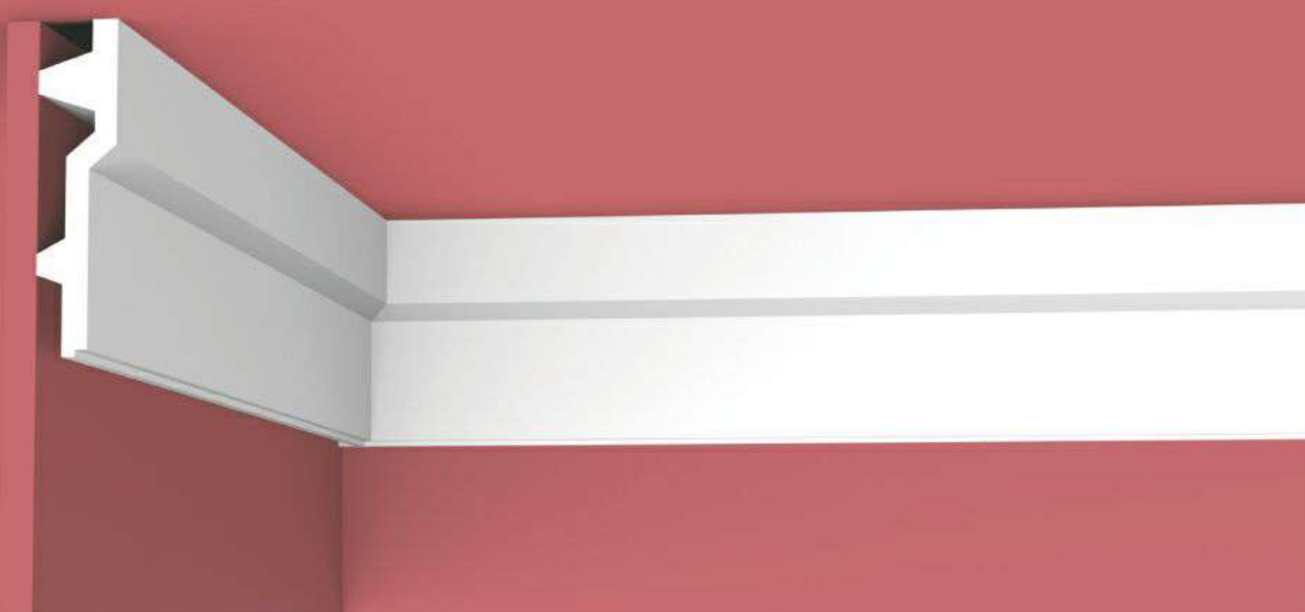
XT-9318 Height x Width x Length 高度 x 宽度 x 长度 180 x 45 x 2400 mm 180 = 180mm 45 180
