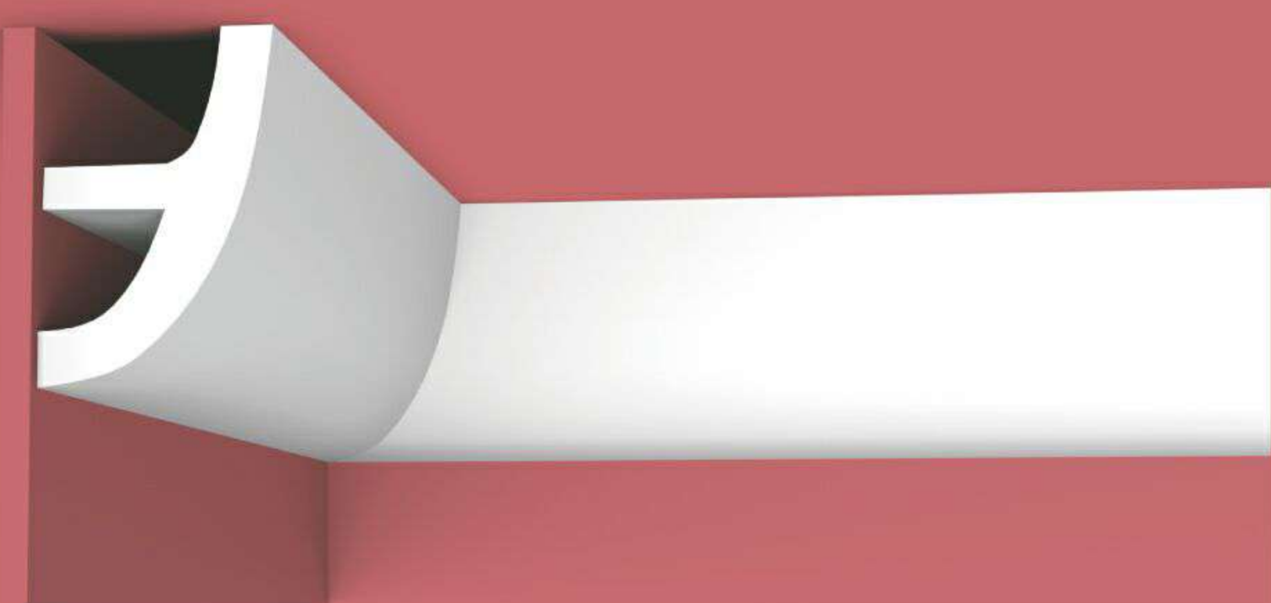
XT-9355 Height x Width x Length 高度 x 宽度 x 长度 80 x 50 x 2400 mm 50 80 95 mm
