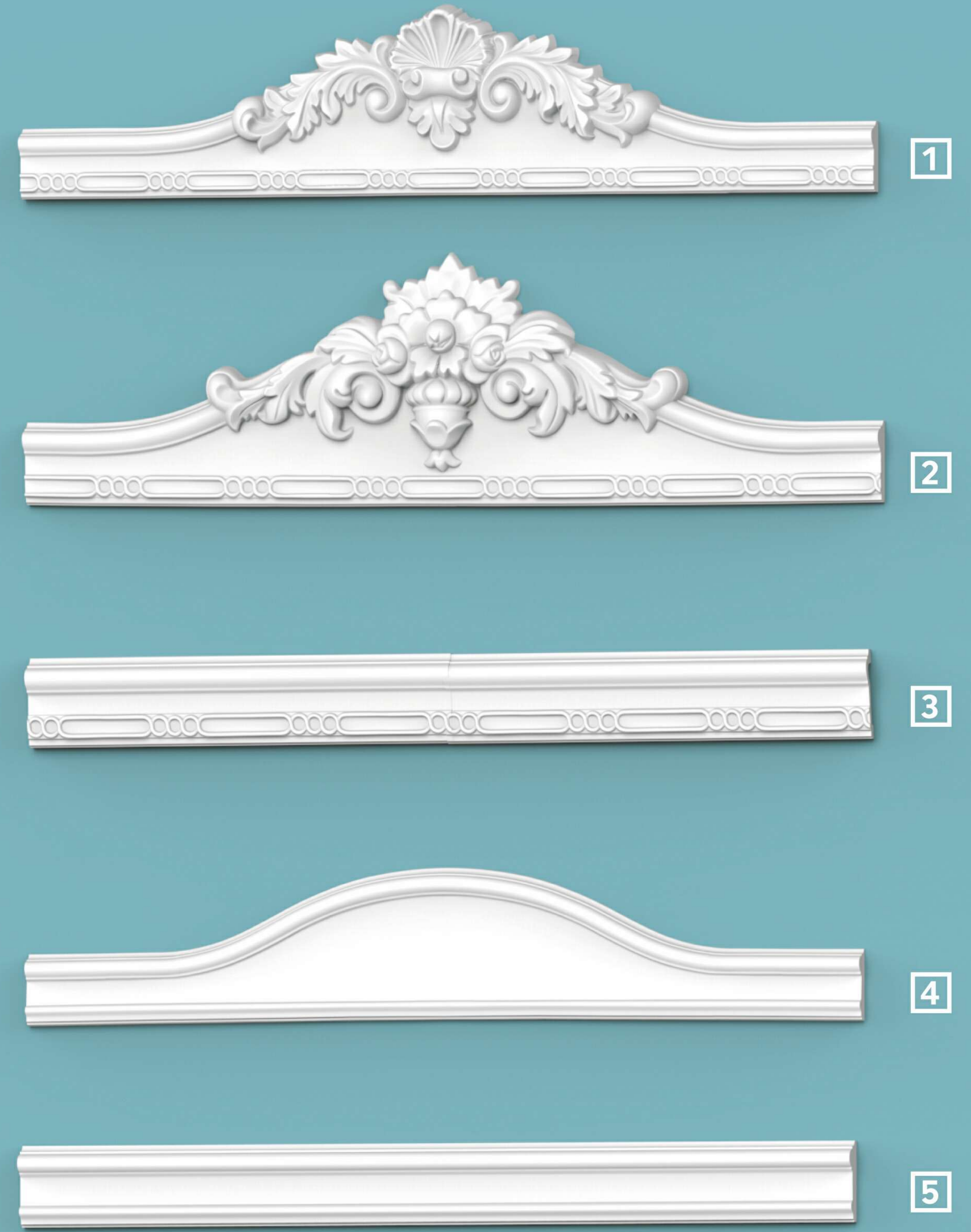
1 XT-9619B Height x Width x Thick 高度 x 宽度 x 厚度 245 x 1250 x 70 mm
