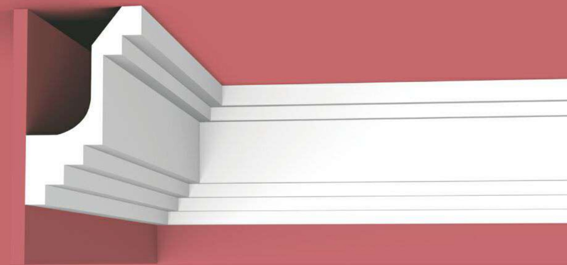
XT-9325 Height x Width x Length 高度 x 宽度 x 长度 100 x 60 x 2400 mm 100 = 117mm 60 100
