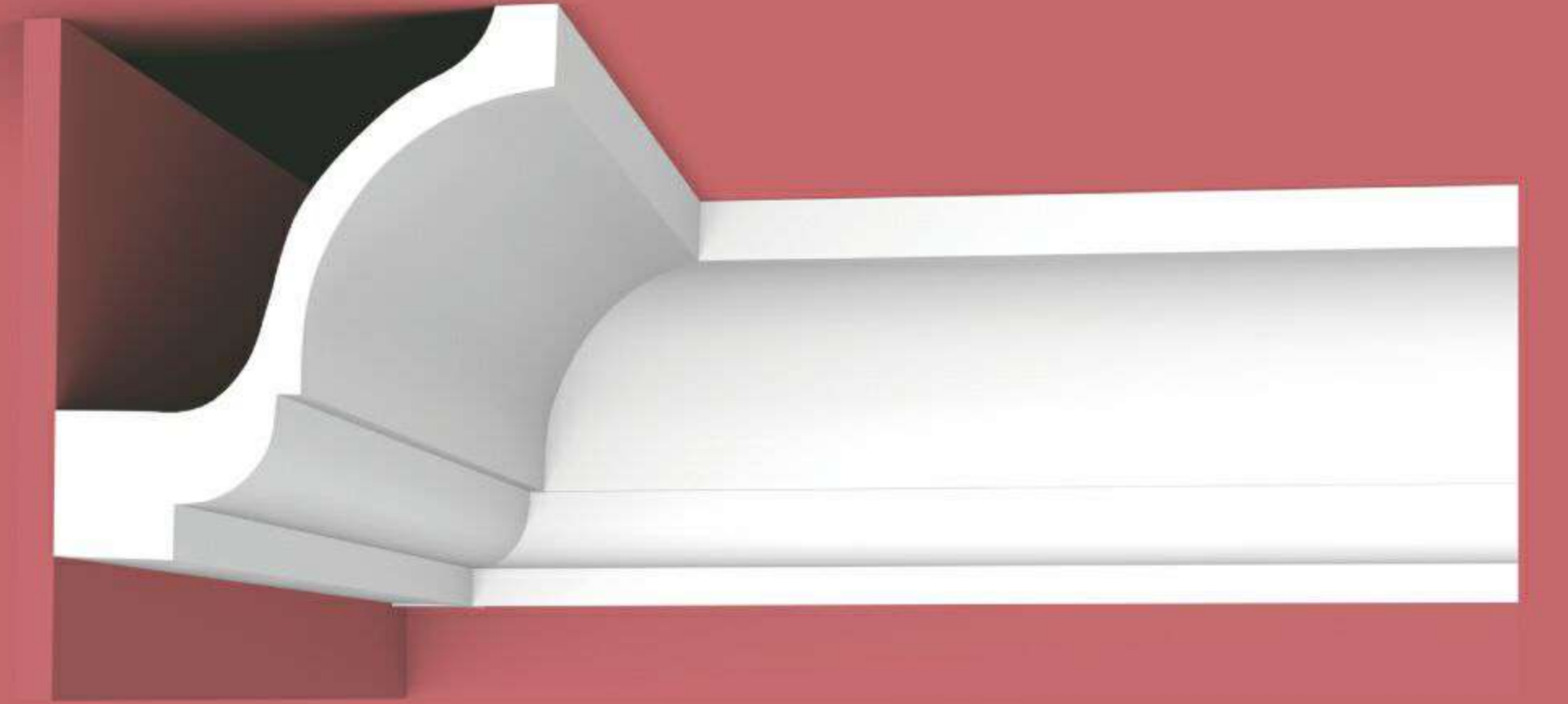
XT-93102 Height x Width x Length 高度 x 宽度 x 长度 138 x 121 x 2400 mm 7 = 180 mm
