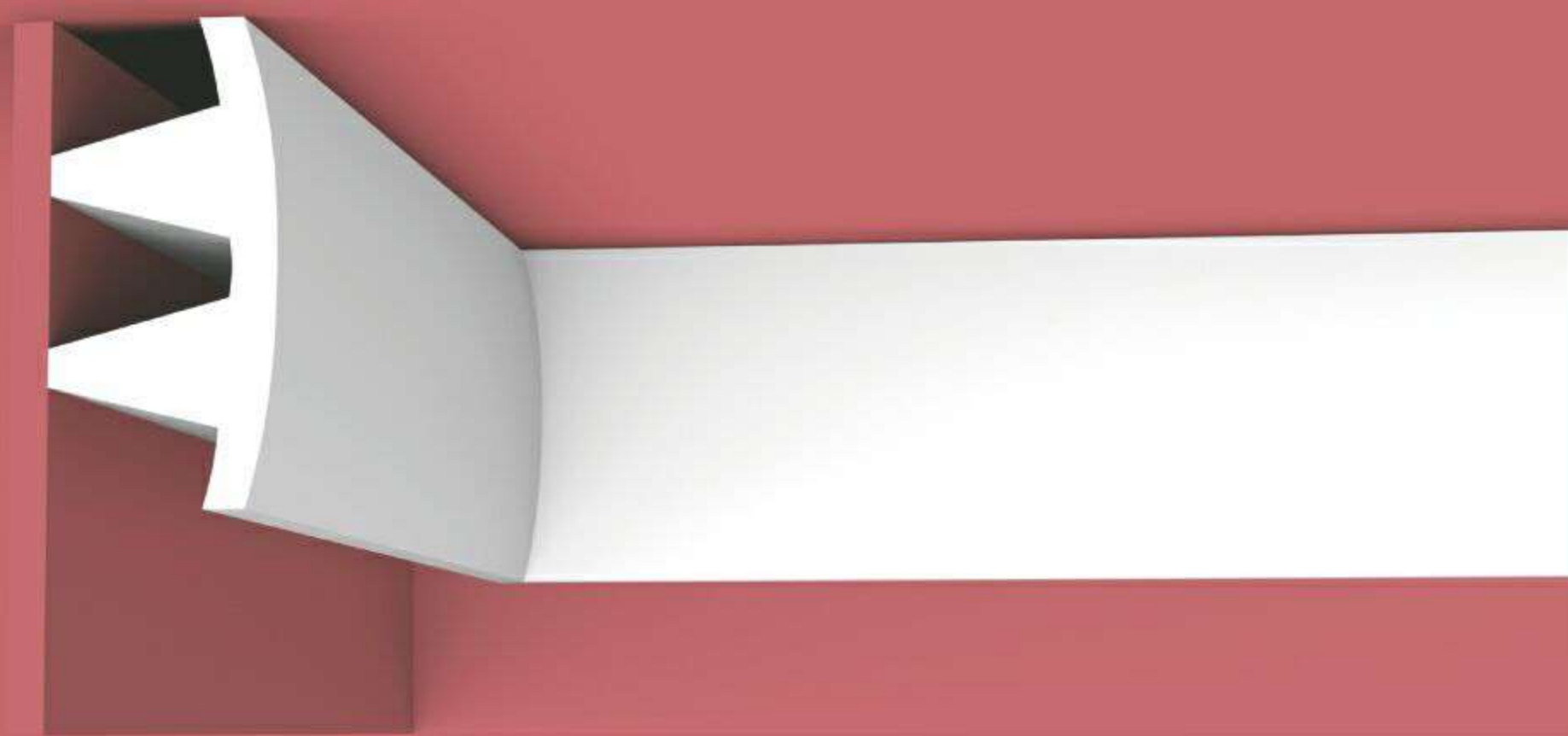
XT-9314 Height x Width x Length 高度 x 宽度 x 长度 100 x 45 x 2400 mm 100 = 110mm 45 100
