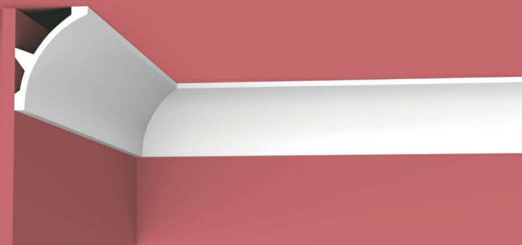
XT-9315 Height x Width x Length 高度 x 宽度 x 长度 140 x 105 x 2400 mm 140 = 175mm 105 140
