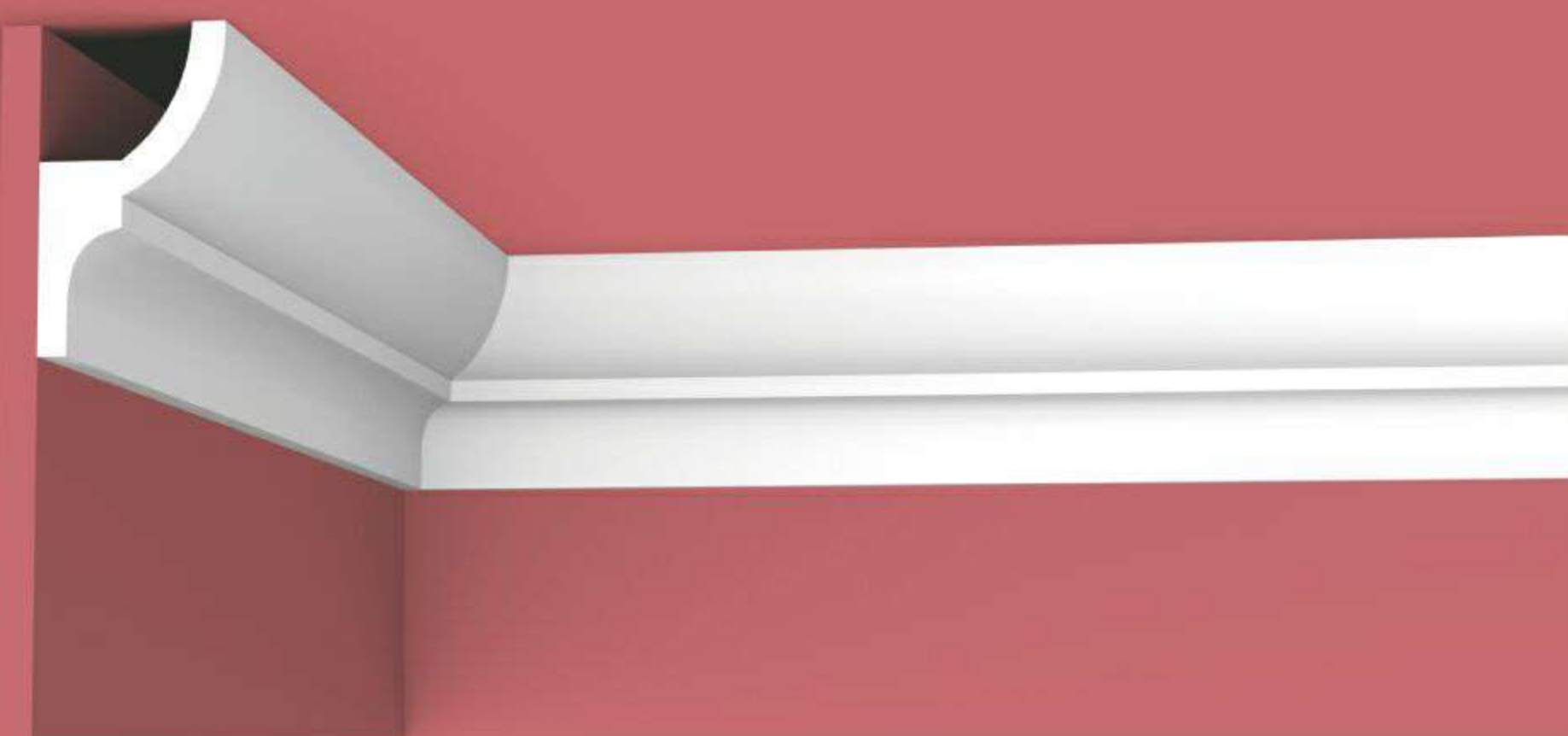
XT-9316 Height x Width x Length 高度 x 宽度 x 长度 70 x 40 x 2400 mm 70 = 81mm 40 70
